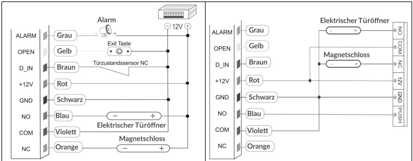
Abb. 1 Standard-Schaltplan
