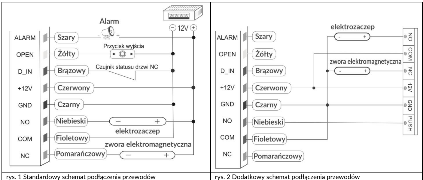
rys. 1 Standardowy schemat podłączenia przewodów
